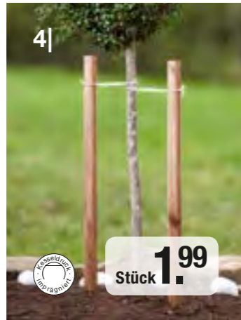
4| MR. GARDENER Pflanzstab Kiefer/Fichte, teakbraun imprägniert. Einseitig angespitzt. Maße Ca. 3 cm Ø, 150 cm lang hbm-Nr. 886248 45619999 Preis Stück 1.99
